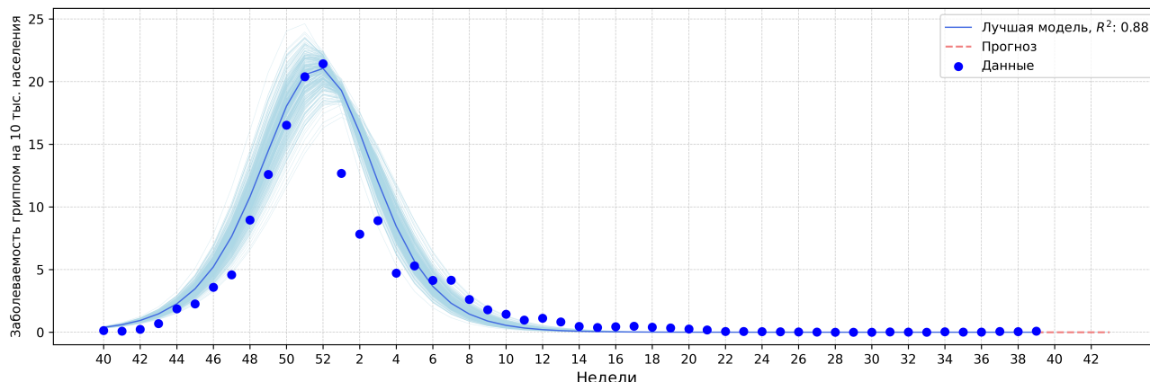
Рис. 13. Результаты моделирования заболеваемости гриппом с начала сезона по 39 неделю 2026г.
